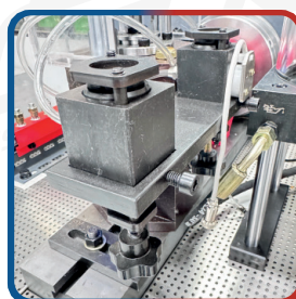
SUPORTE UNIVERSAL 2 INJETORES
